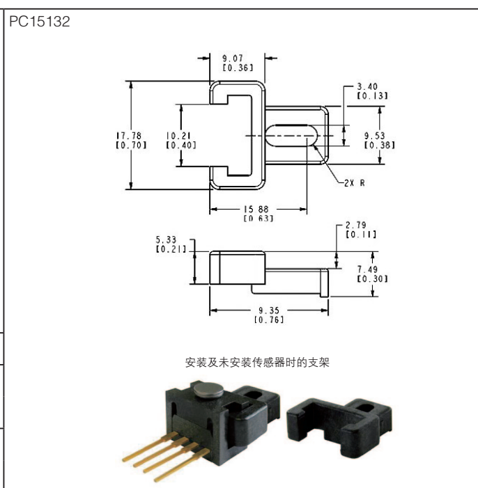
图 3：塑料安装支架安装尺寸图（仅供参考：mm/[in]）
