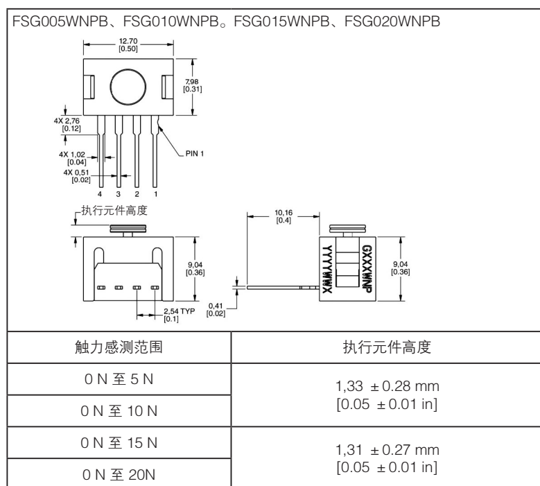
图 2：传感器安装尺寸（仅供参考：mm/[in]）
